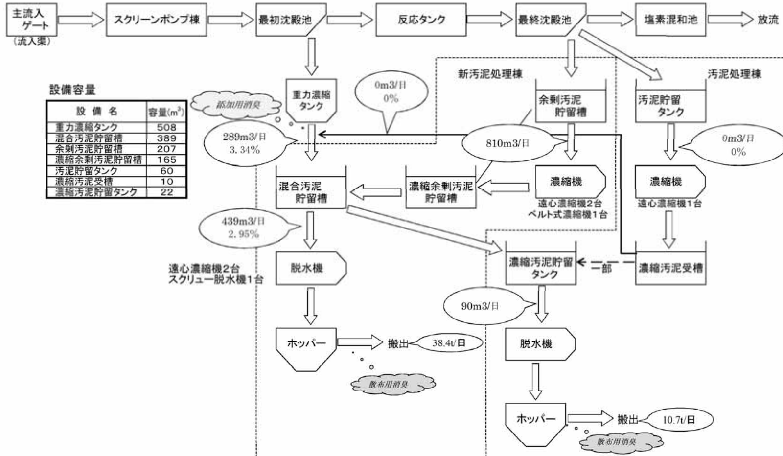
汚泥処理状況（平成25年1月平均）
