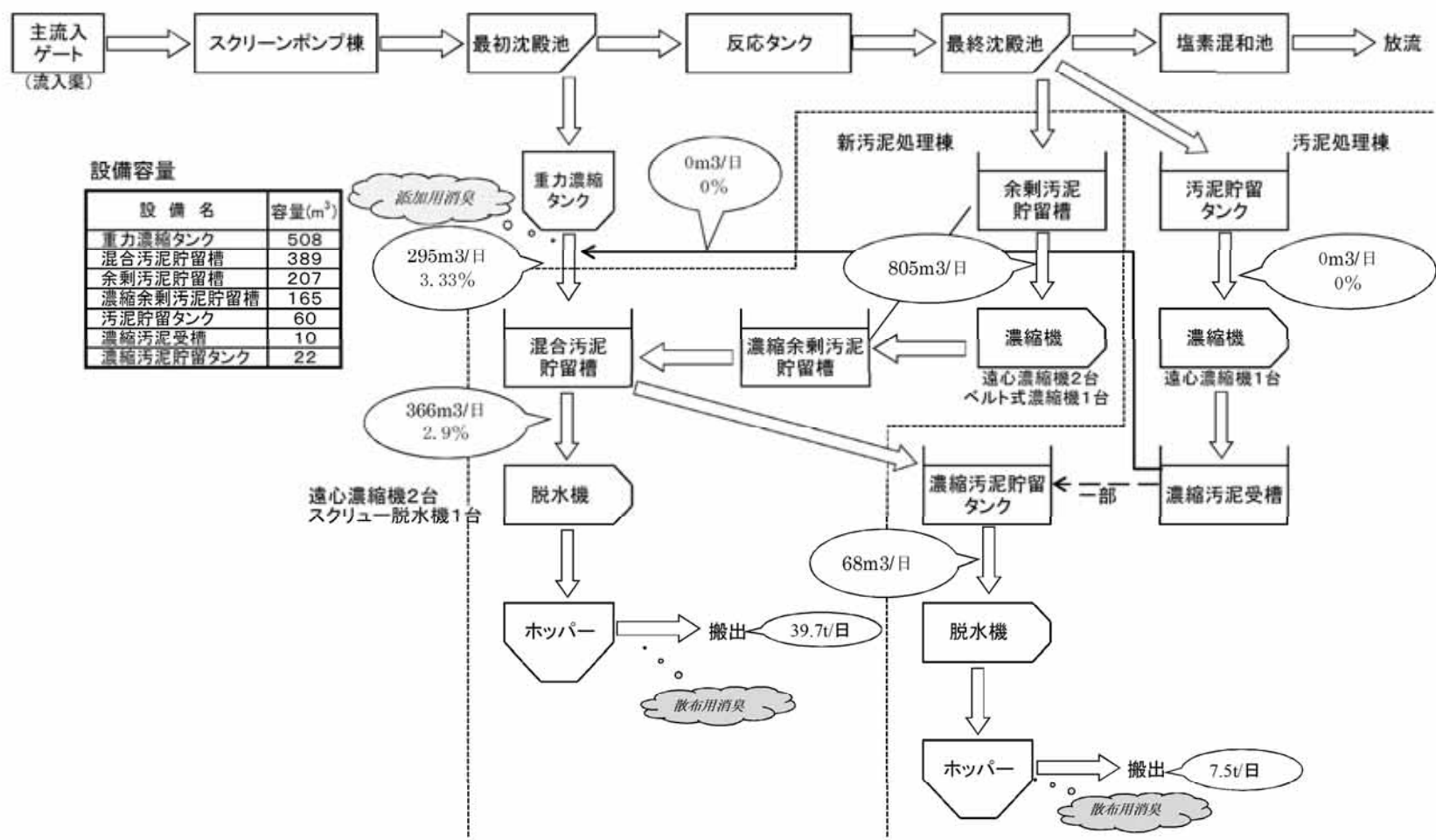
汚泥処理状況（平成24年1月平均）
