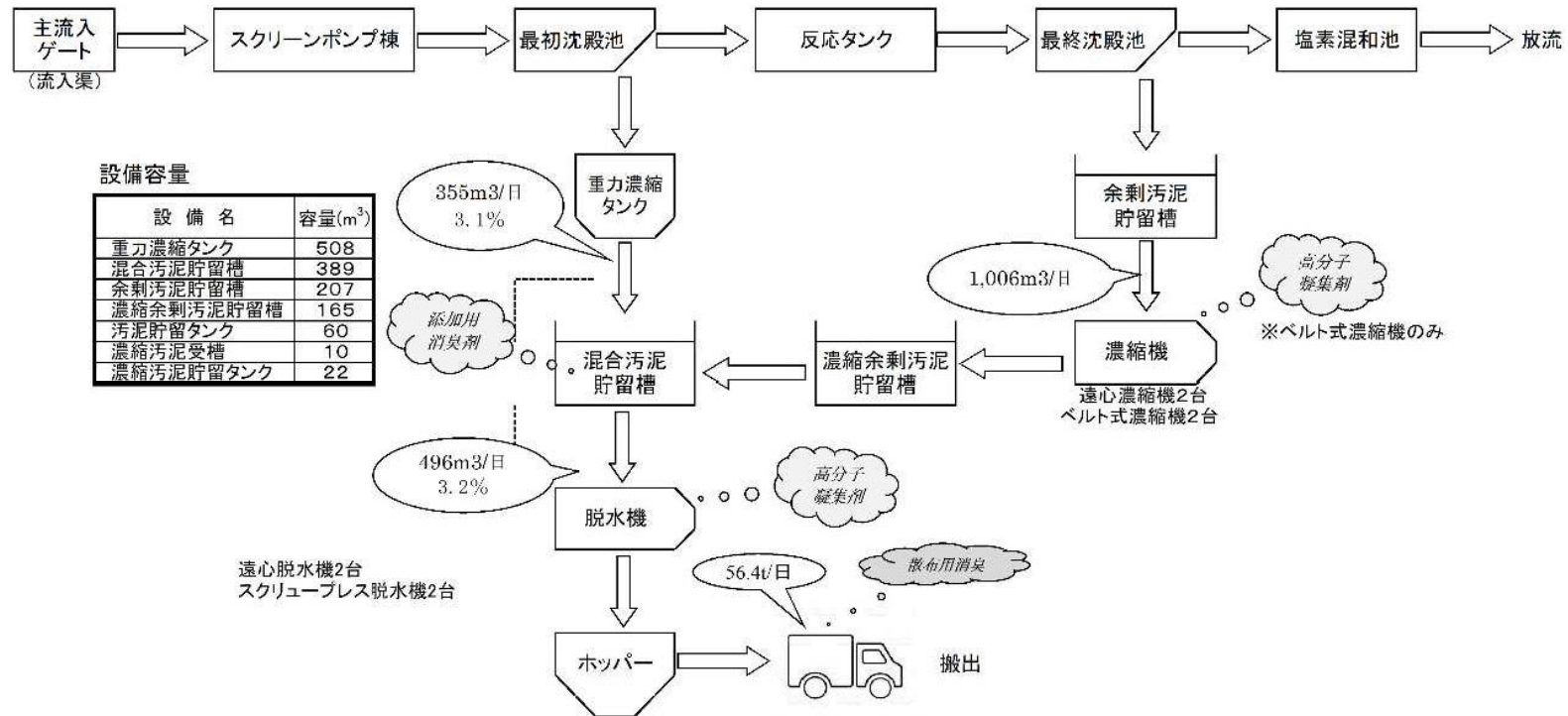
汚泥処理状況（令和5年12月平均）
