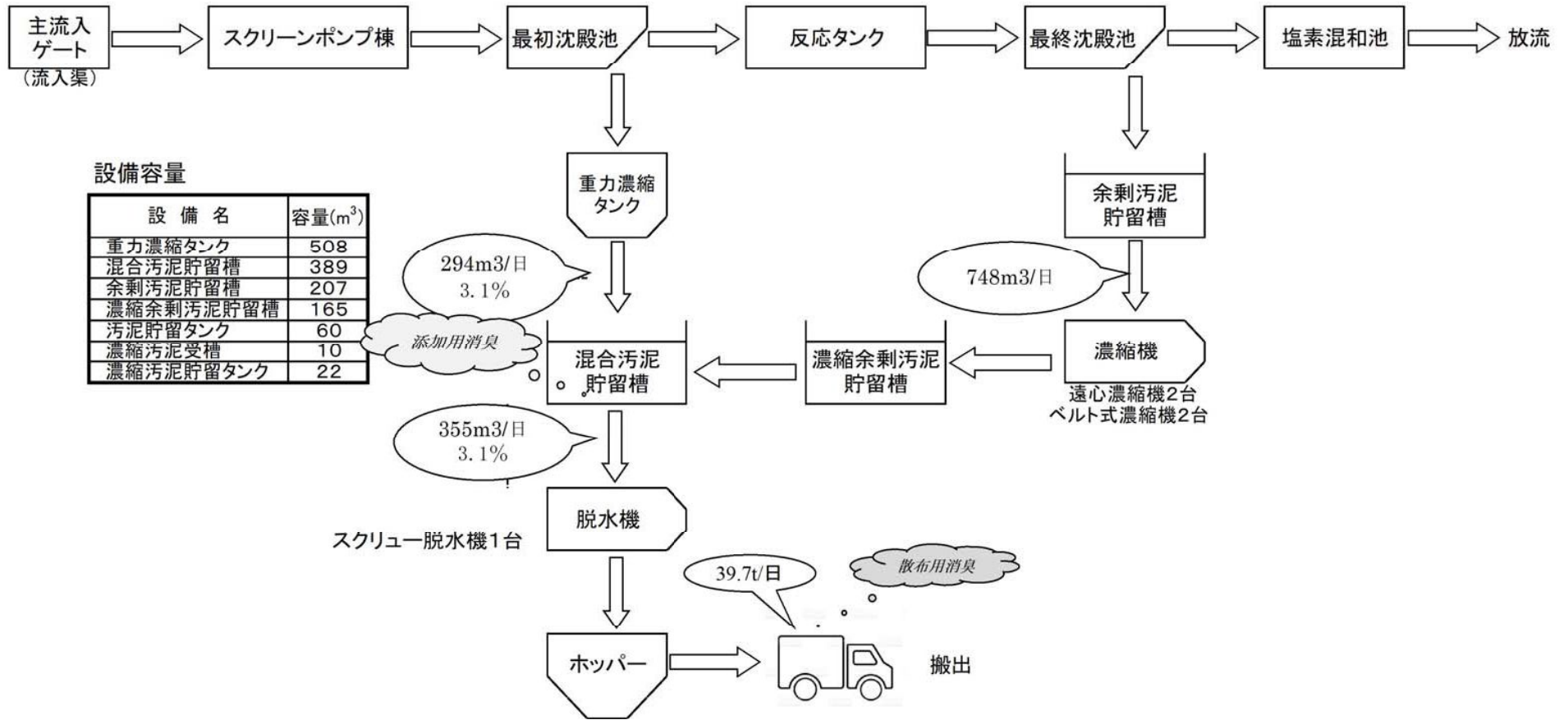
汚泥処理状況（令和3年12月平均）
