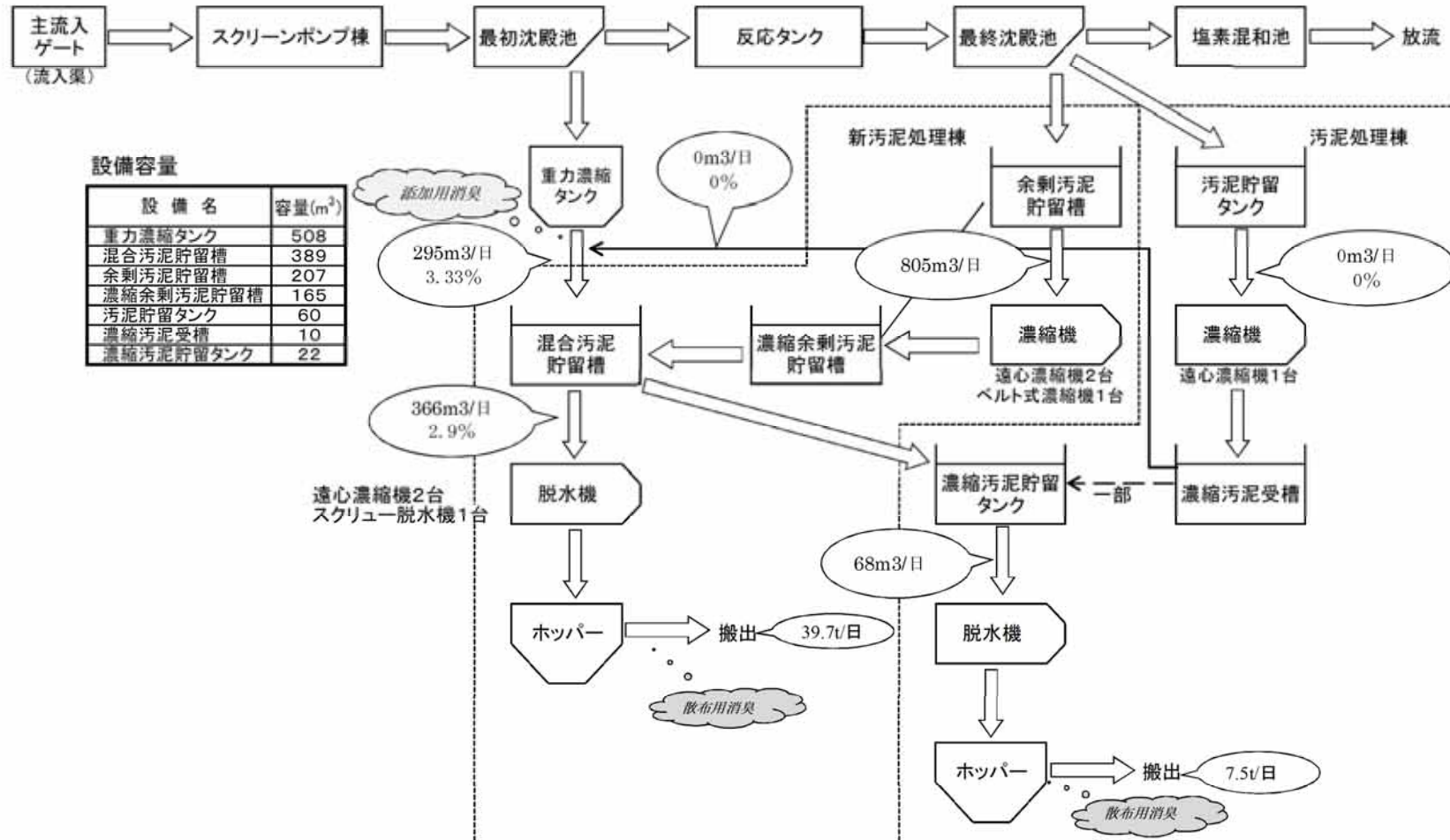
汚泥処理状況（平成24年1月平均）
